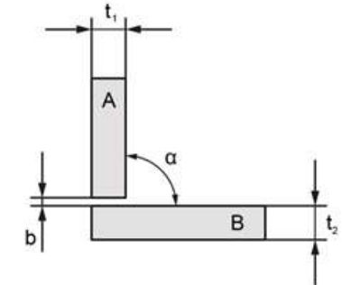
Hoeklas, pijp-pijp
